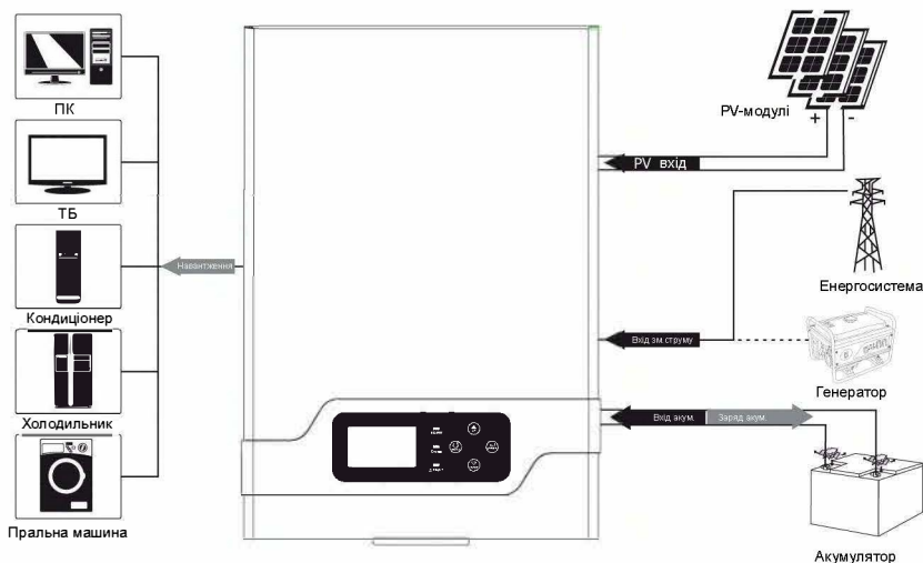
мал.1 Гібридна система живлення
